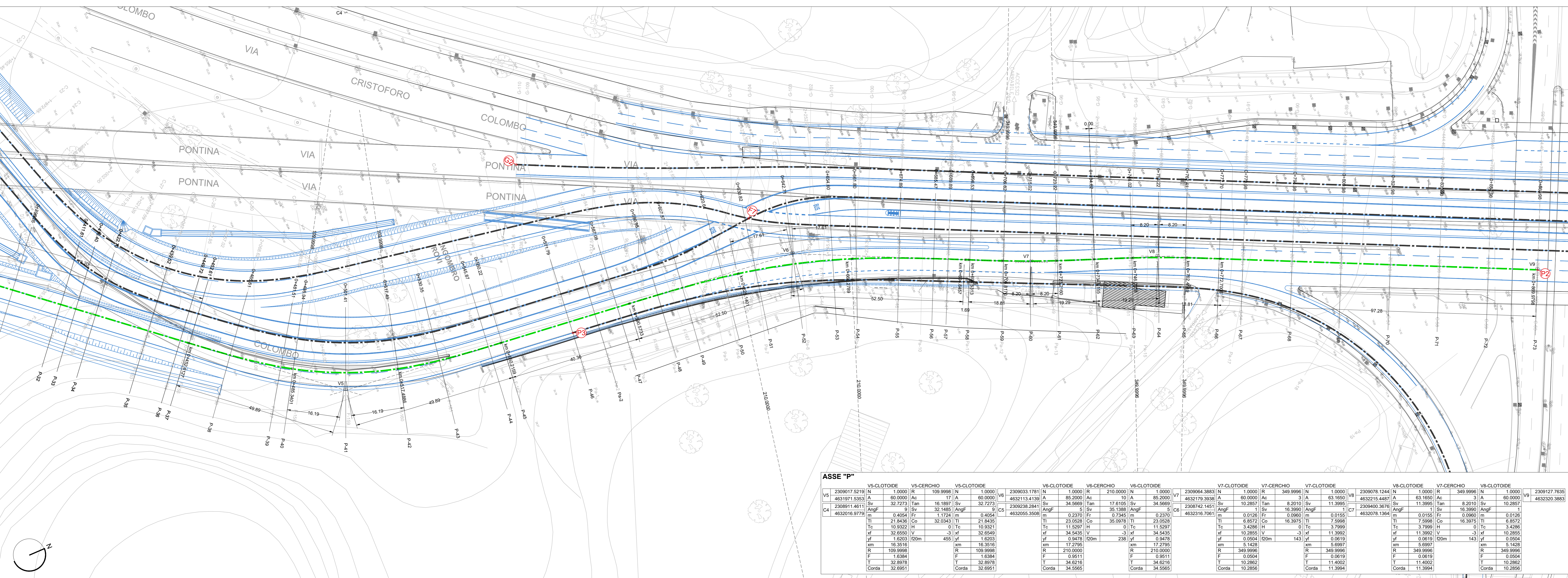
PLANIMETRIA DI TRACCIAMENTO - ASSE PONTINA DIR. EUR ("P") da prog. Km 0+411.61 a prog. Km 0+869.98
