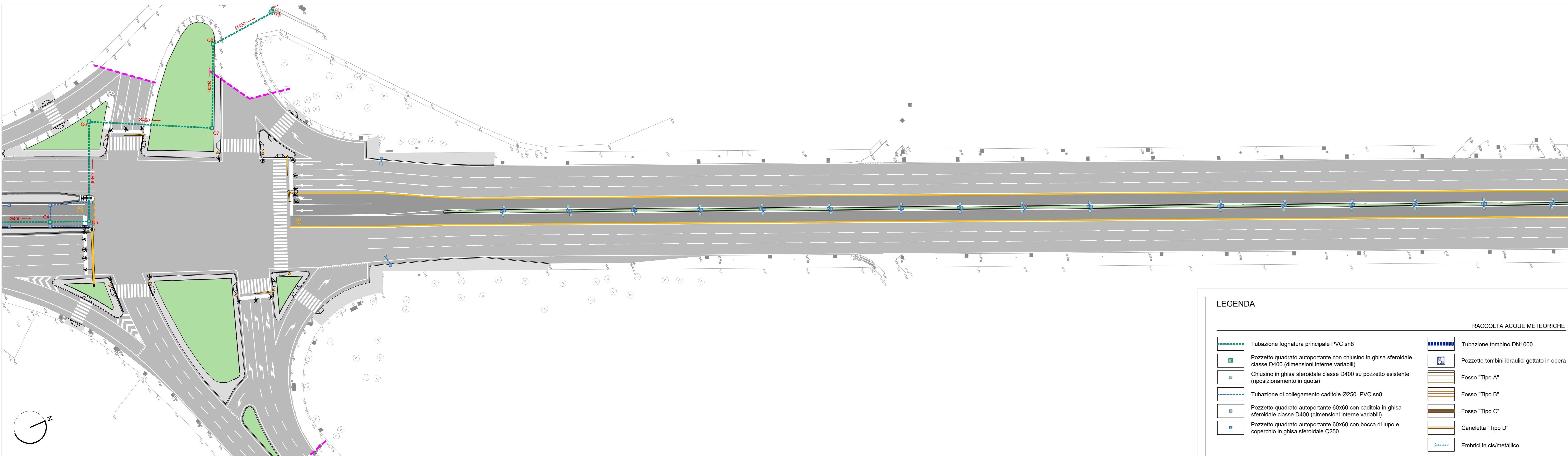
PLANIMETRIA SMALTIMENTO ACQUE DI PIATTAFORMA - da Piazza 25 Marzo 1957 a via Algeria
