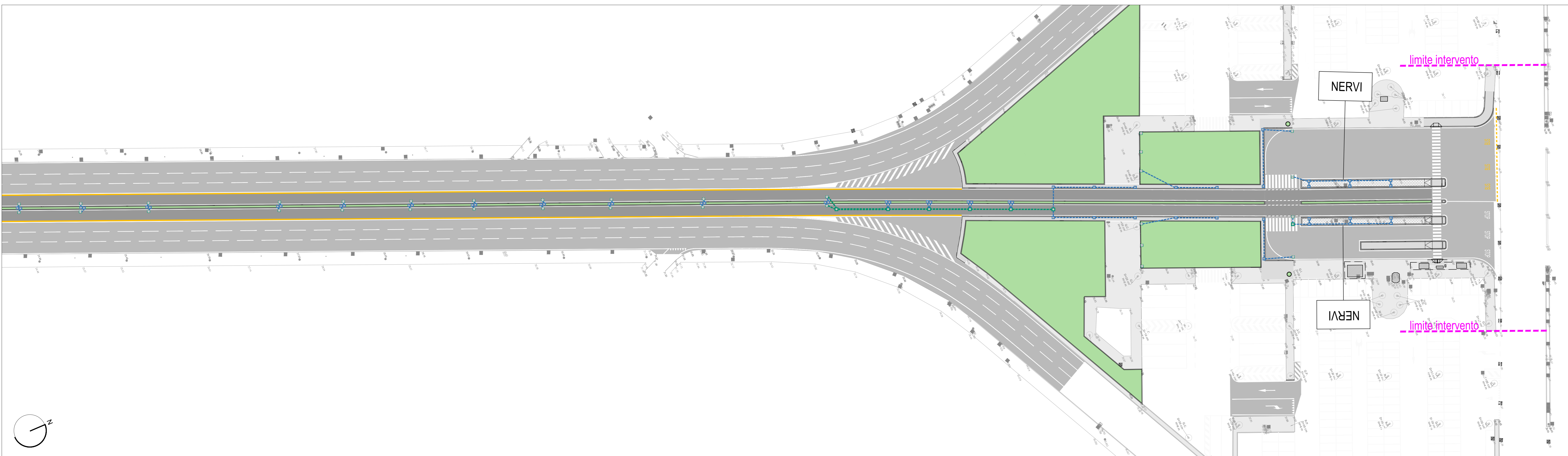
PLANIMETRIA SMALTIMENTO ACQUE DI PIATTAFORMA - da via Algeria a Piazzale Nervi
